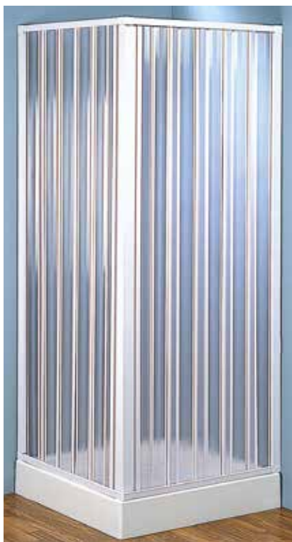
cabina doccia a soffietto 100% PVC stabilizzato, binario metrato per una facile riduzione di larghezza, h 185 cm 80x80 cm - 110x110 cm optional: terza parete
